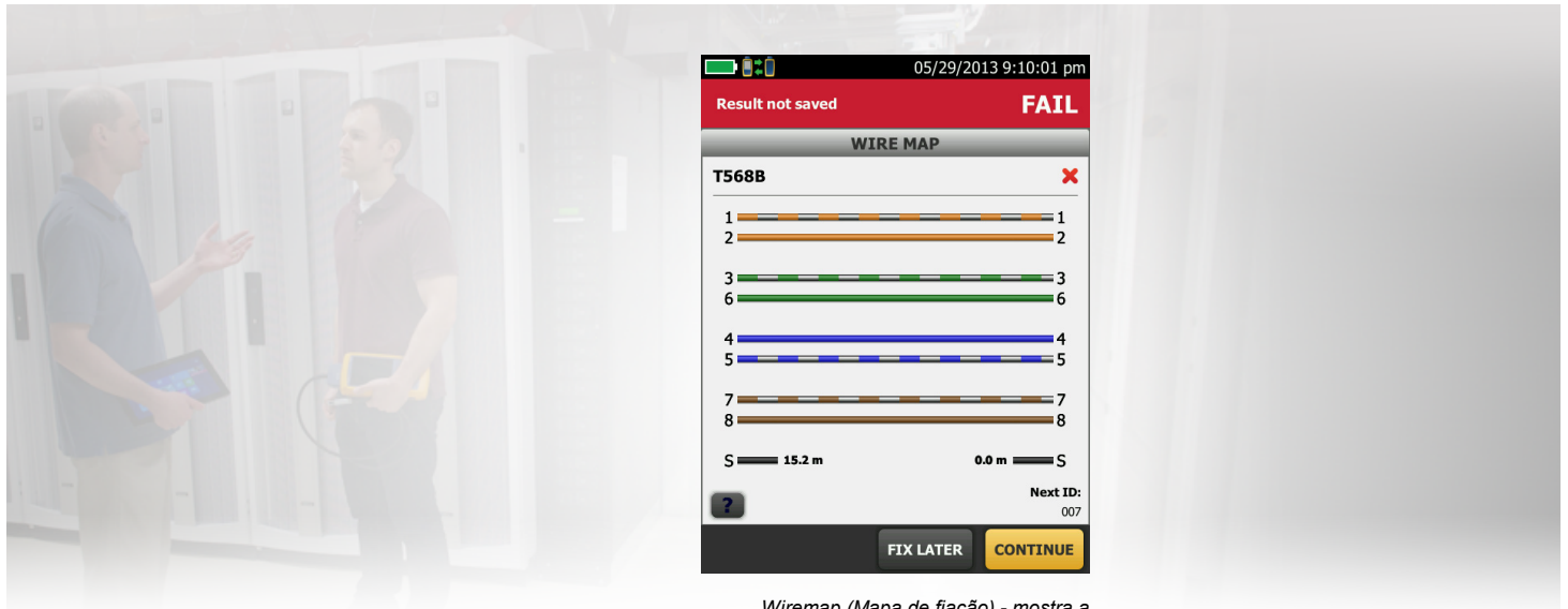
Wiremap (Mapa de fiação) - mostra a distância até a falha, ruptura e falta
